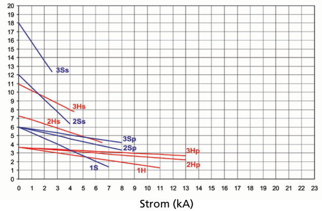
Hochstromausgang - ODEN AT Systeme für 240 V, 50 Hz
